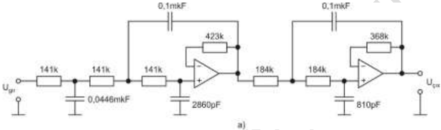
Şəkil 1. Beşsıra saylı süzğəci
