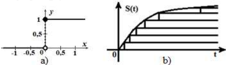
Şəkil 2. a) Hevisaydın vahid funksiyası; b) siqnalın dinamik təqdim olunması
