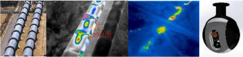
Şəkil. Adi və termal kamera vasitəsilə neft-qaz kəmərlərinin analiz görüntüləri
