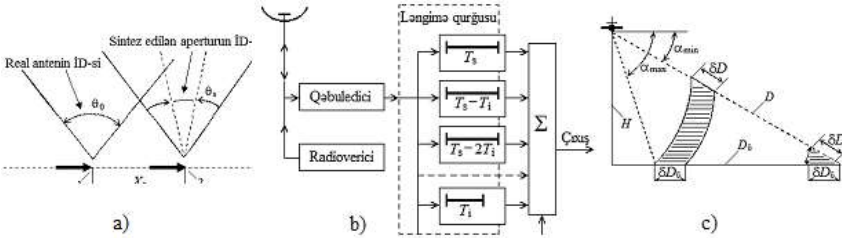
Şəkil 1. a) sintez edilən İD; b) SARL-ın struktur sxemi; c) ayırdetmənin təyini prinsipi
