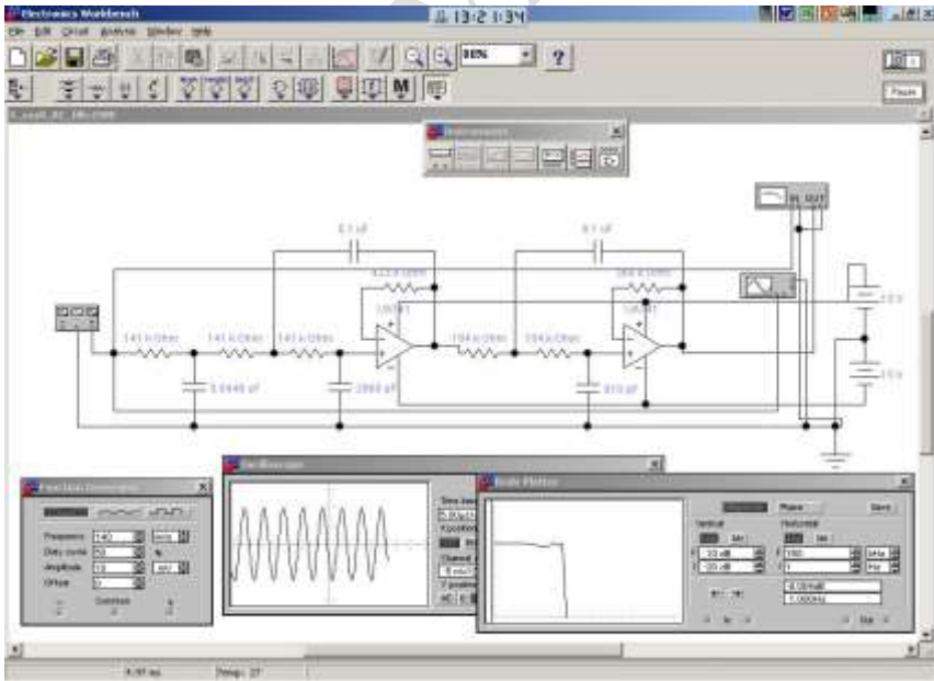
Şəkil 2. Beşsıra saylı süzğəcin sxeminin tədqiqi
