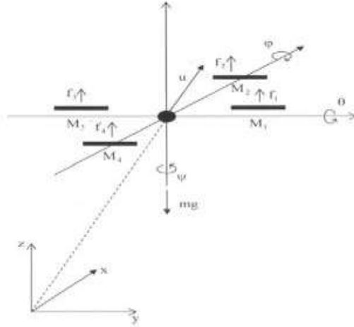
Şəkil 1. Kvadrokopterin sxemi
