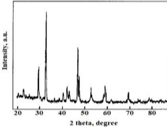
Şəkil 1. \text{Nd}_{0.5}\text{Sr}_{0.5}\text{MnO}_3 birləşməsinin rentgen difraksiyası spektri
