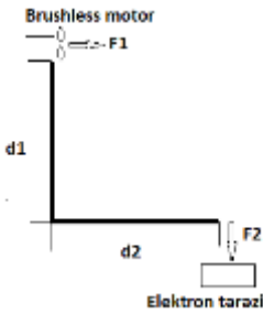
Şəkil 1. Fırçasız motorları test etmək üçün stendin sxemi və görünüşü
